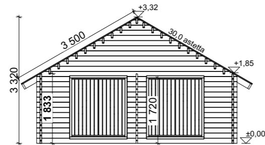
Snitt 1:100
