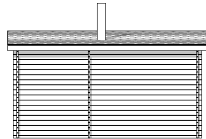
Fasad 1:100
