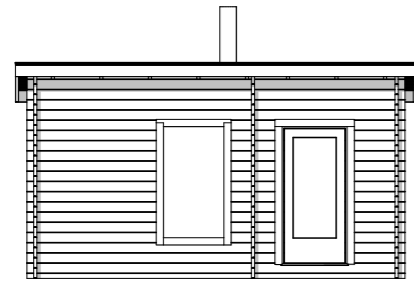
Fasad 1:100
