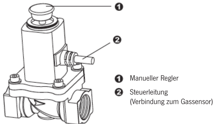
Elektromagnetisches Ventil (optionales Zubehör)
