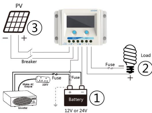
Kuva 3 Kytentäkaavio
