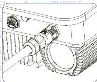
Figur 6.3 Snabbkopplingschema för växelström
