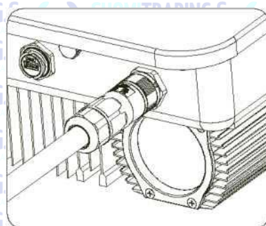
Kuva 6.3 Vaihtovirran pikaliitännäkaavio
