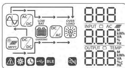
Kuva 22: LCD-näytön symbolit
