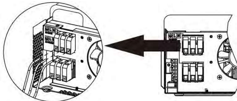
Kuva 7: AC-tulon kytkentä
