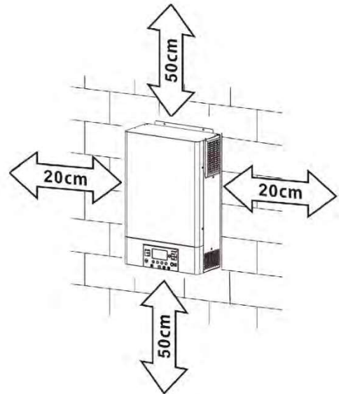
Kuva 5.1: Minimisuojaetäisyydet
