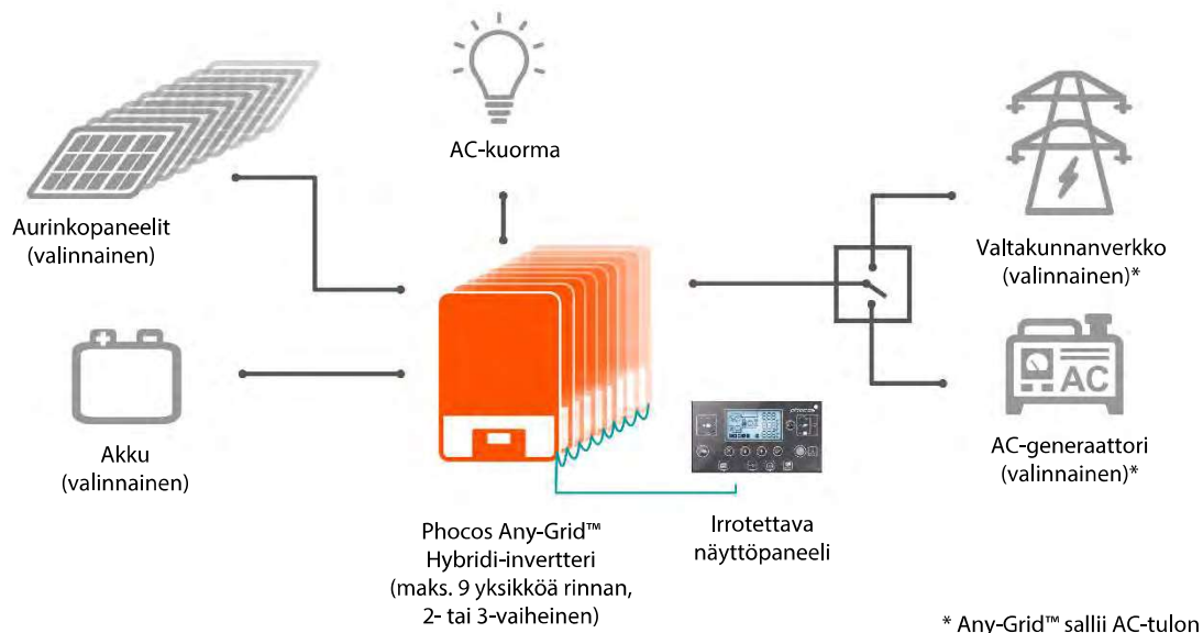
Kuva 1: Järjestelmä
