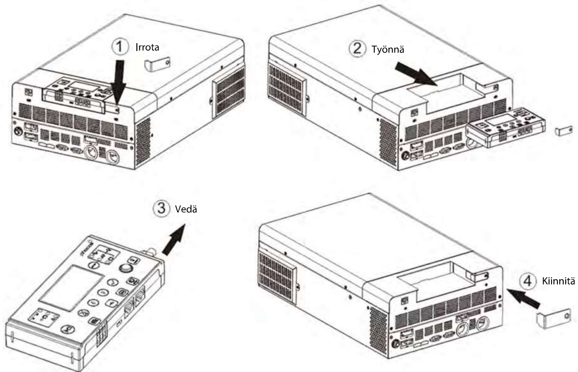
Kuva 11: Näyttöpaneelin irrottaminen
